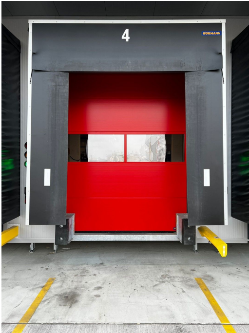
Hörmann Verladerampe-HTL-2 mit einem Industrie-Sektionaltor-SPU F42
